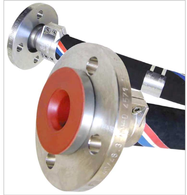
PFA-beschichtete Schlaucharmaturen. FEP schlauch
