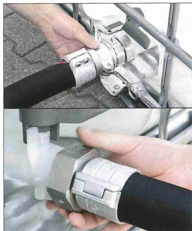
Reduzierstück (oben) und Mutterteil-Schlauchverschraubung
