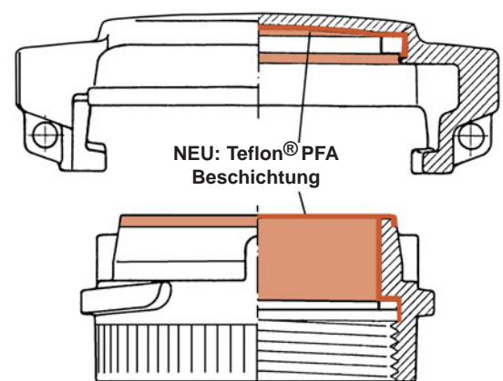
Beispiel: Type VK ...SSE
